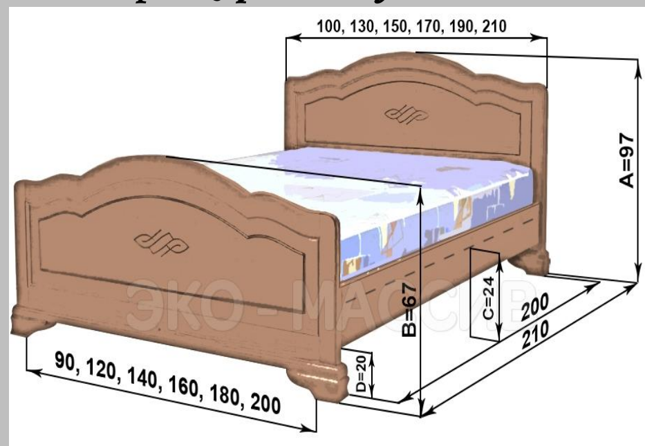
Чертеж кровати Муза
