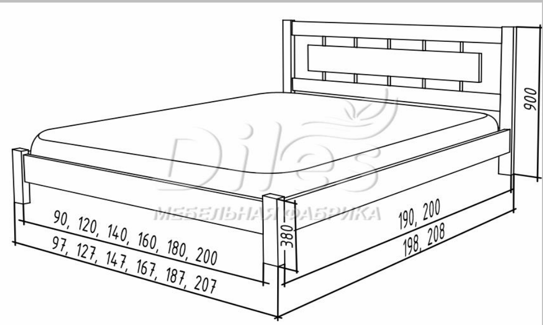
Чертеж кровати Сакура
