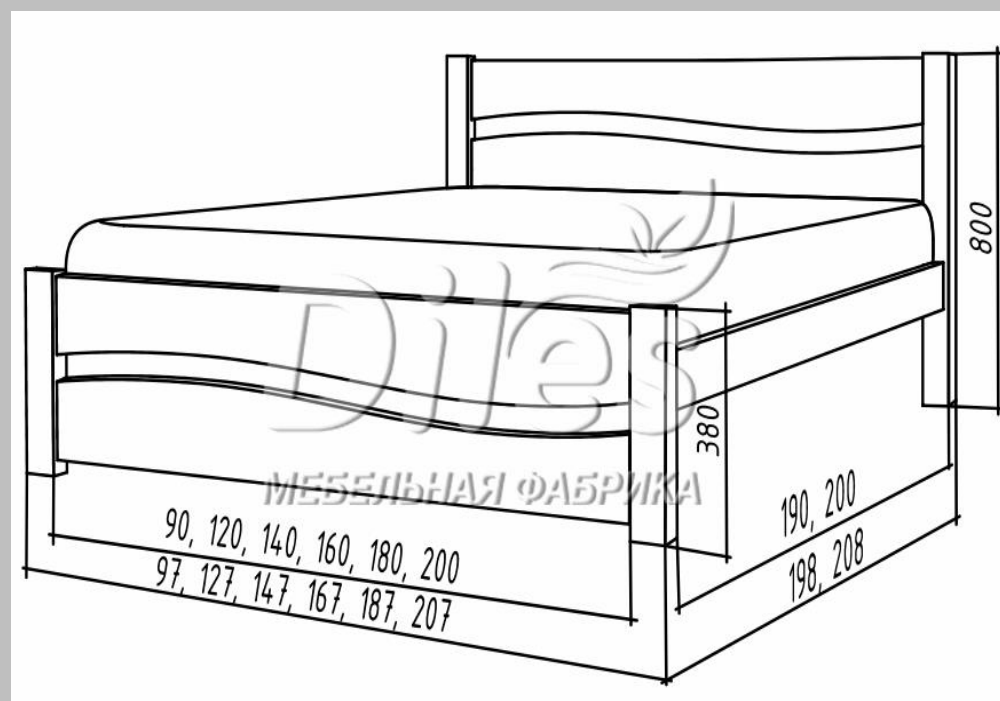
Чертеж кровати Волна
