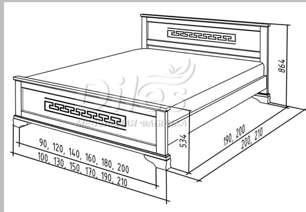
Чертеж кровати Афина
