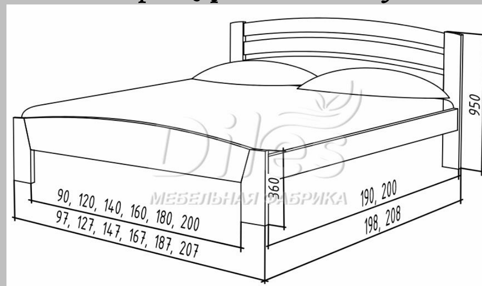
Чертеж кровати Селена гнутая
